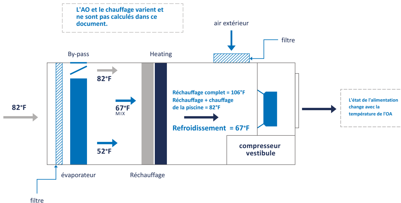
FIGURE 20 : DÉSHUMIDIFICATEURS PAR RÉFRIGÉRATION
