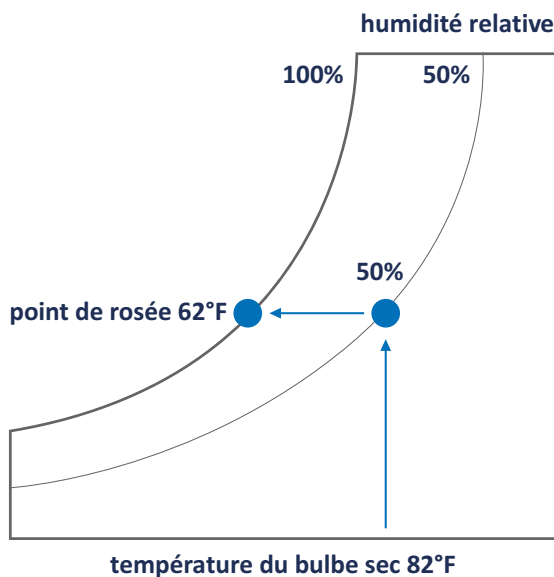
FIGURE 4 : TEMPÉRATURE DU POINT DE ROSÉE
