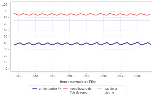
FIGURE 18 : LE SERPENTIN DE RÉCHAUFFAGE À GAZ CHAUD ENTRAÎNE DES TEMPÉRATURES ET DES NIVEAUX D'HUMIDITÉ RELATIVE INSTABLES
