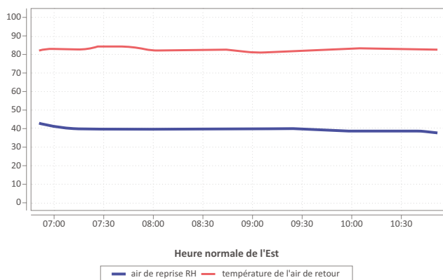
FIGURE 19 : LE SYSTÈME DE RÉCHAUFFAGE MODULANT DE SERESCO FOURNIT DES TEMPÉRATURES ET DES NIVEAUX D'HUMIDITÉ RELATIVE STABLES. ET DES NIVEAUX D'HUMIDITÉ RELATIVE STABLES
