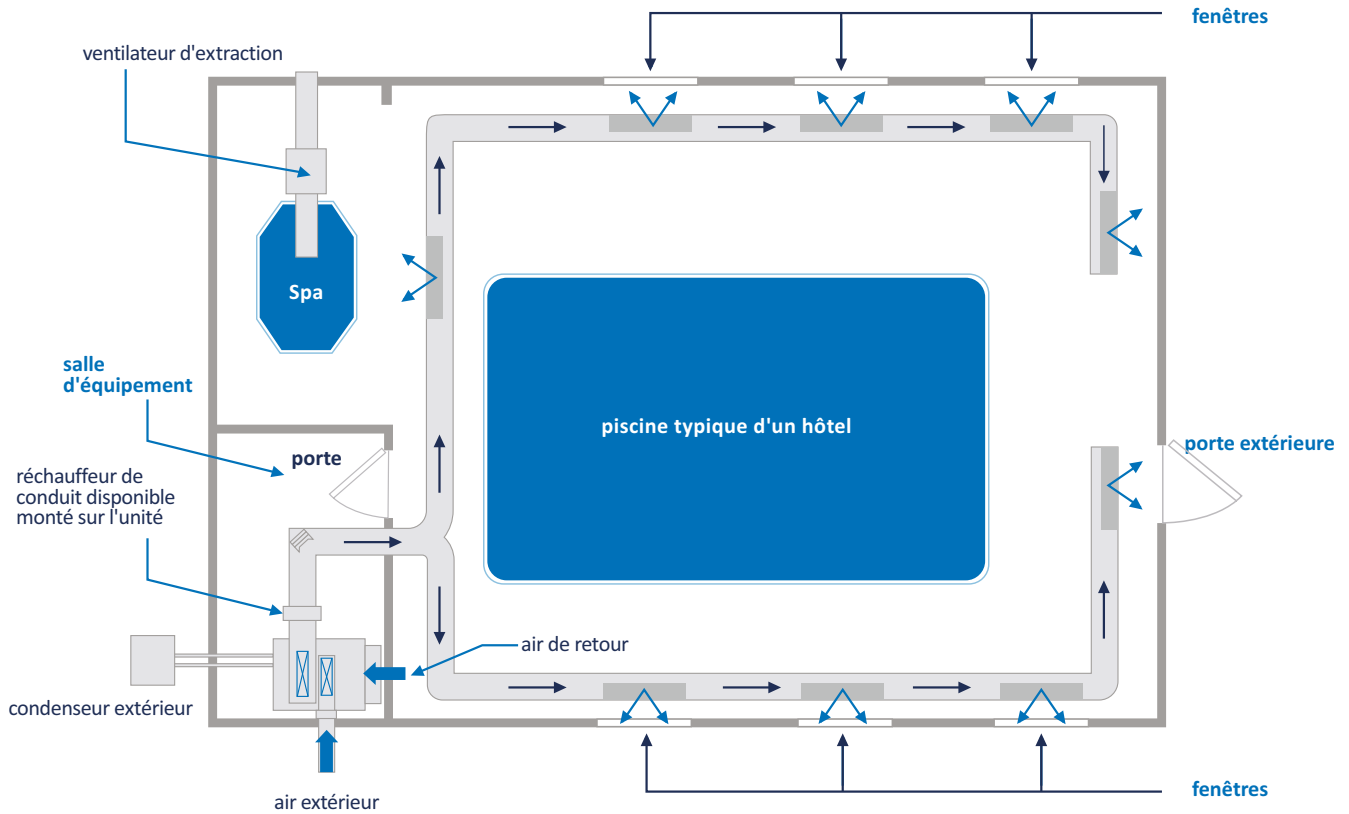
FIGURE I3 : DISPOSITION TYPIQUE D'UN HÔTEL ET D'UNE PISCINE THÉRAPEUTIQUE
